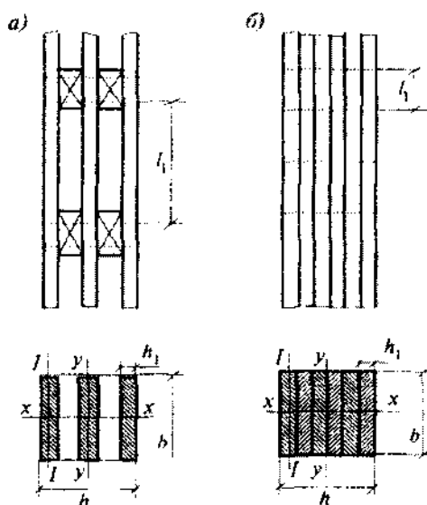
а – с прокладками; б – без прокладок Рисунок 2 - Составные элементы
