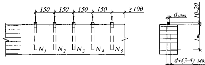
Рисунок И.3 - Схема образцов для испытаний
