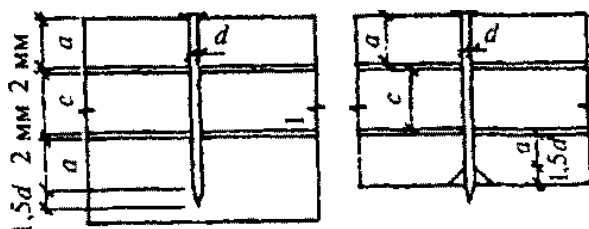
Рисунок 12 - Определение расчетной длины заземления конца гвоздя
