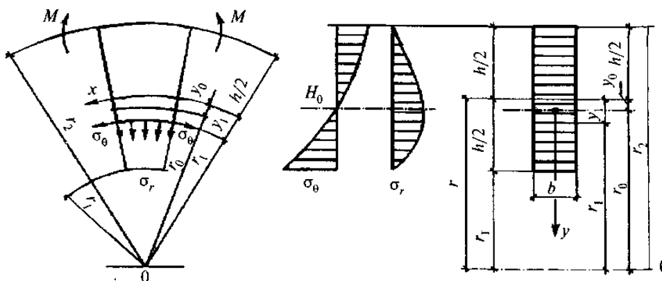
Рисунок 3 - Расчетная схема кривого бруса при чистом изгибе
