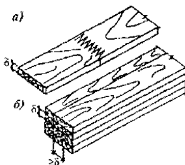
Рисунок 7 - Клеевые соединения
