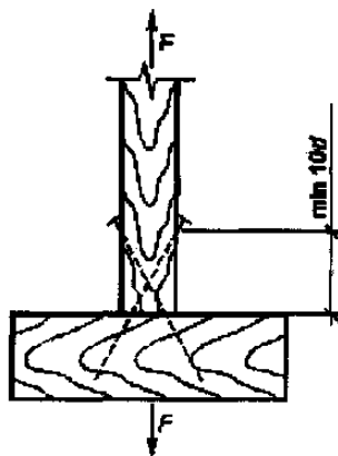
Рисунок 14 - Наклонная забивка гвоздей
