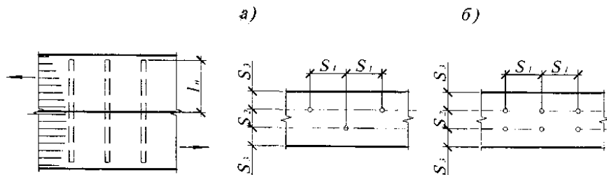
а - шахматная расстановка; б - двухрядная расстановка Рисунок 18 - Соединение на клеенных стальных нагелях
